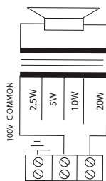
Schaltplan
