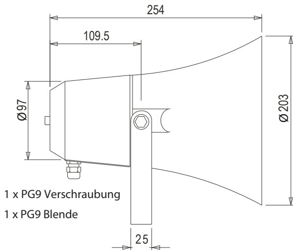
Seitenansicht (Masseinheit: mm)
