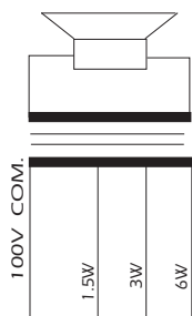
Schéma de branchement
