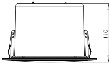
Vue de côté (unité de mesure : mm)
