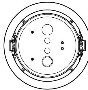
Vue arrière (unité de mesure : mm)
